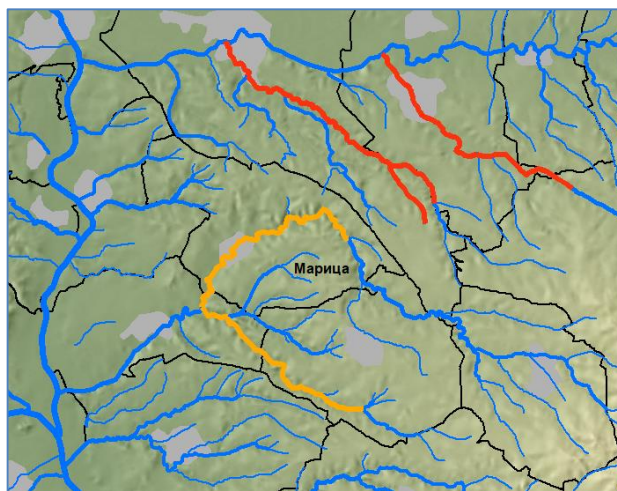
Фигура 2: Правило за обща отточна точка за образуване на РЗПРН
