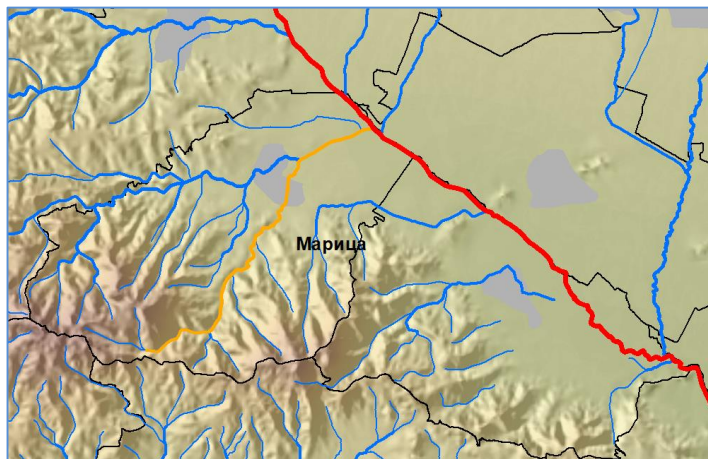
Фигура 3: Правило за особеностите на релефа и формирането на оттока
