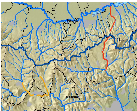
Фигура 1: Правило за разположение на РЗПРН в рамките на един речен басейн.
