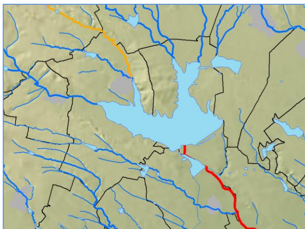
Фигура 4: Правило за комплексни язовири при определянето на РЗПРН
